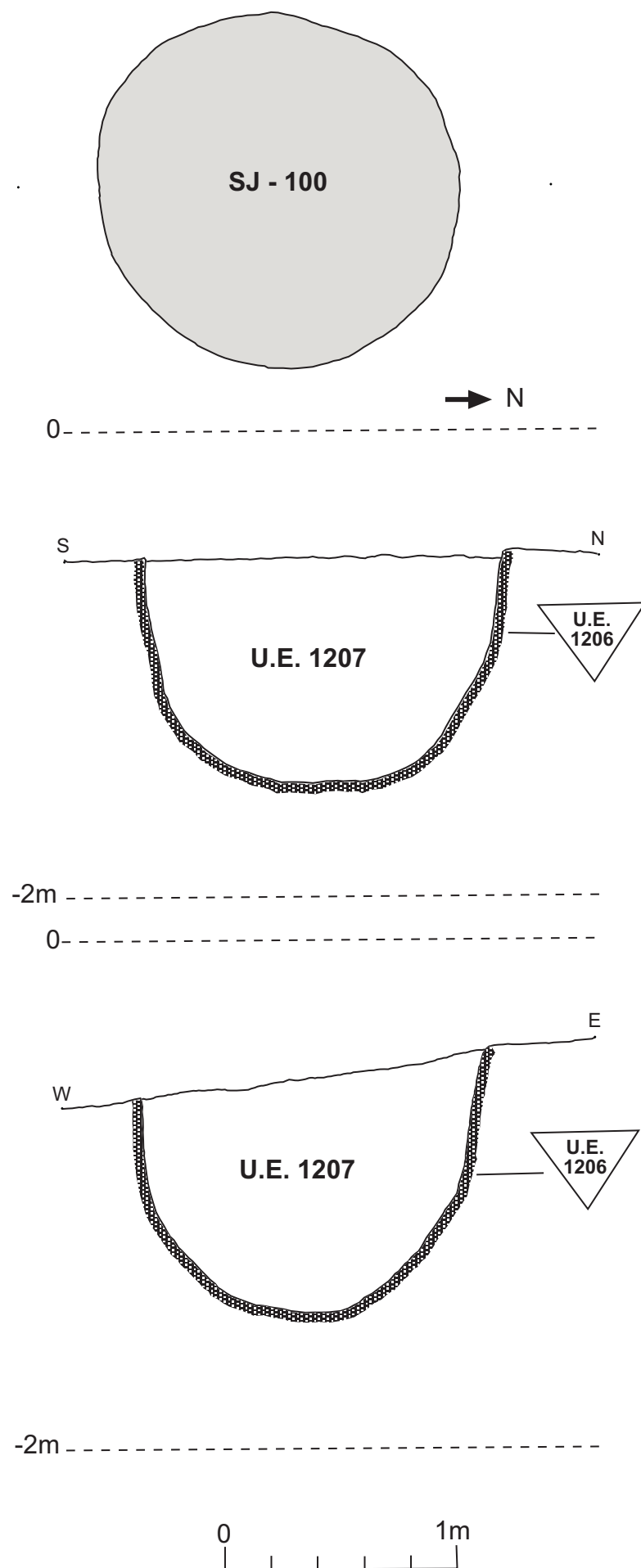
Fig. 11.- Planta i secció de la SJ-100.
