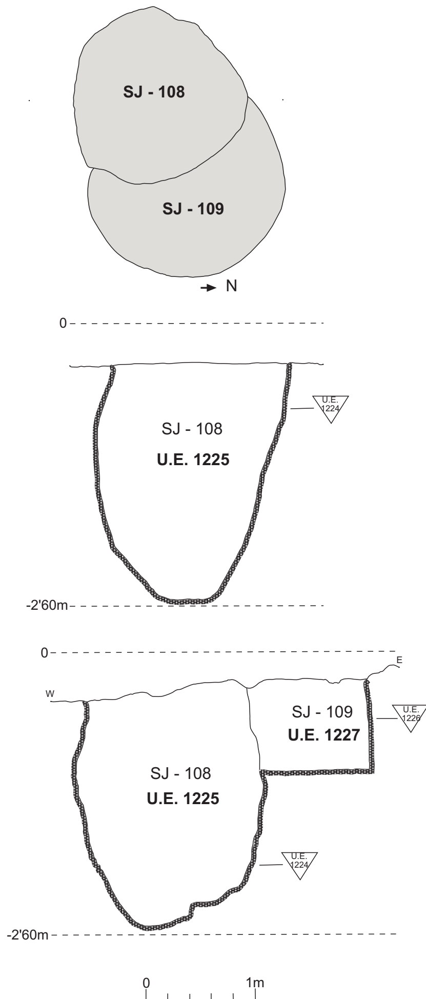
Fig. 23.- Planta i secció de les SJ-108 i SJ-109.
