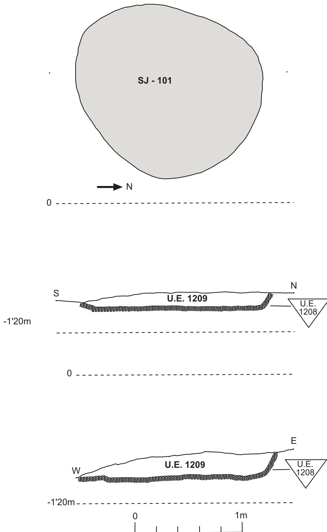
Fig. 13.- Planta i secció de la SJ-101.
