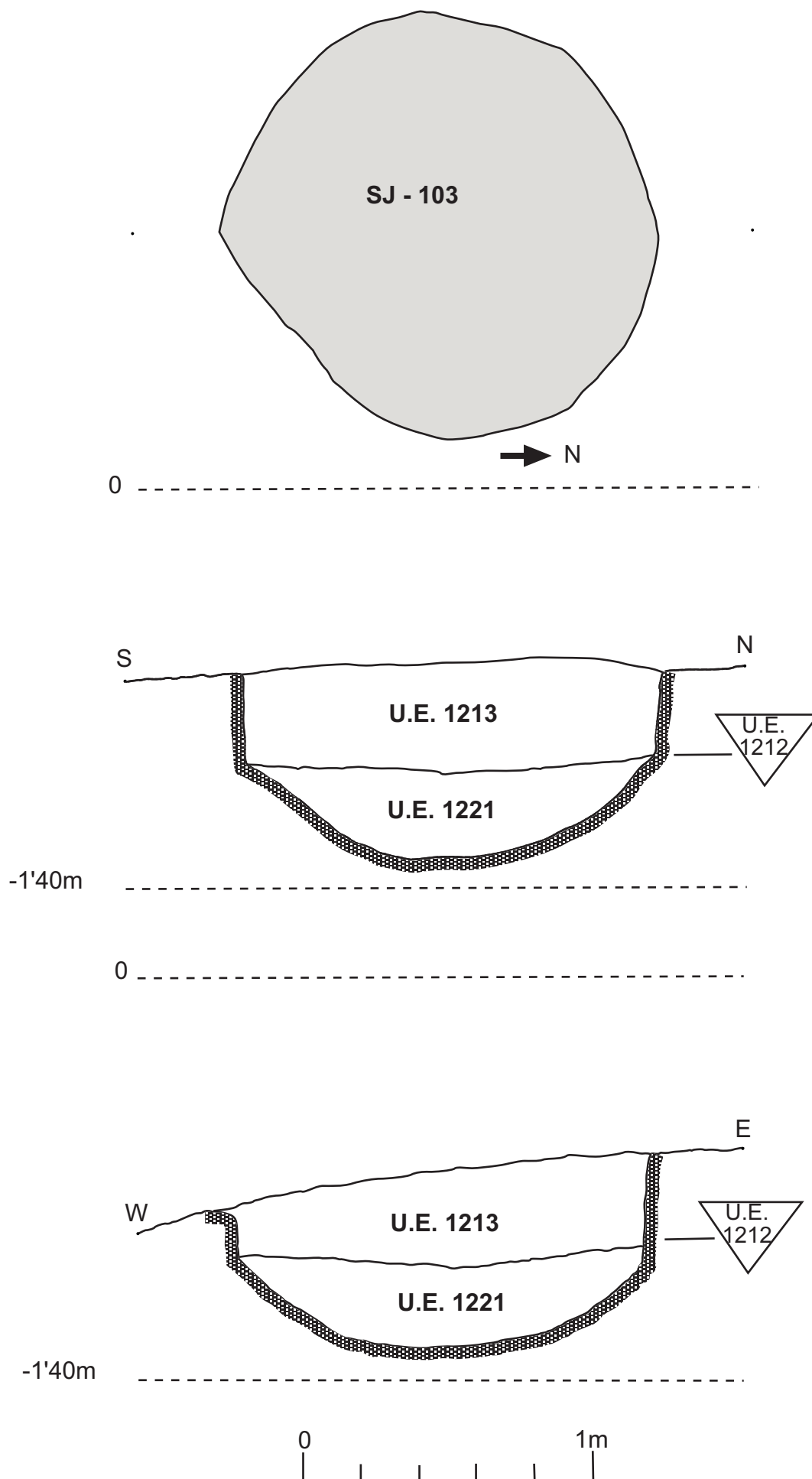
Fig. 17.- Planta i secció de la SJ-103.
