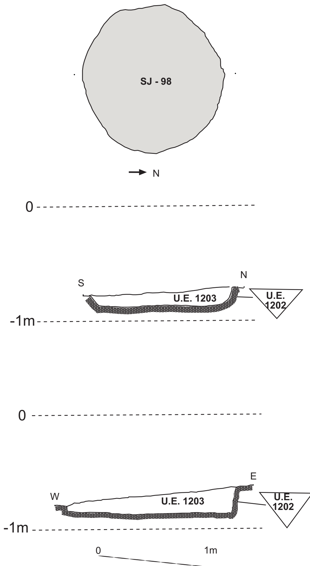
Fig. 7.- Planta i secció de la SJ-98.
