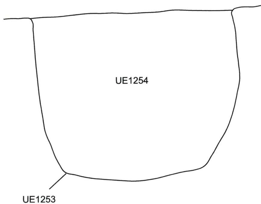
Fig. 4.- Planta i secció de la SJ121.
