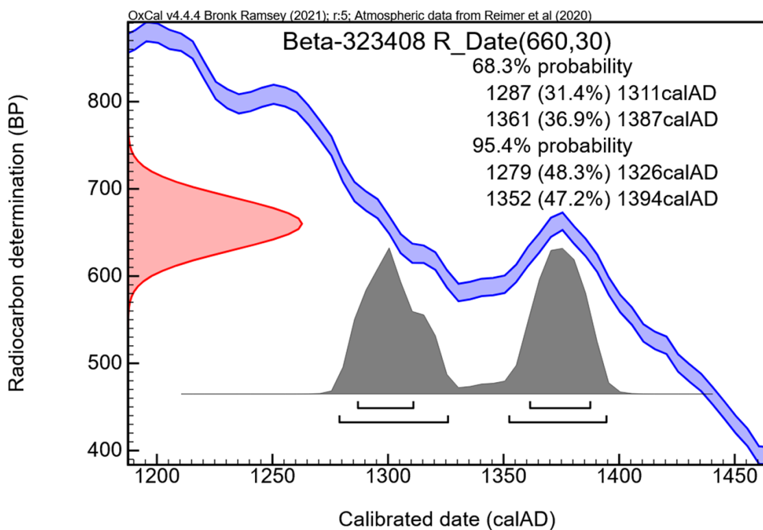
Figura 67. Calibració de la datació BETA-323408.
