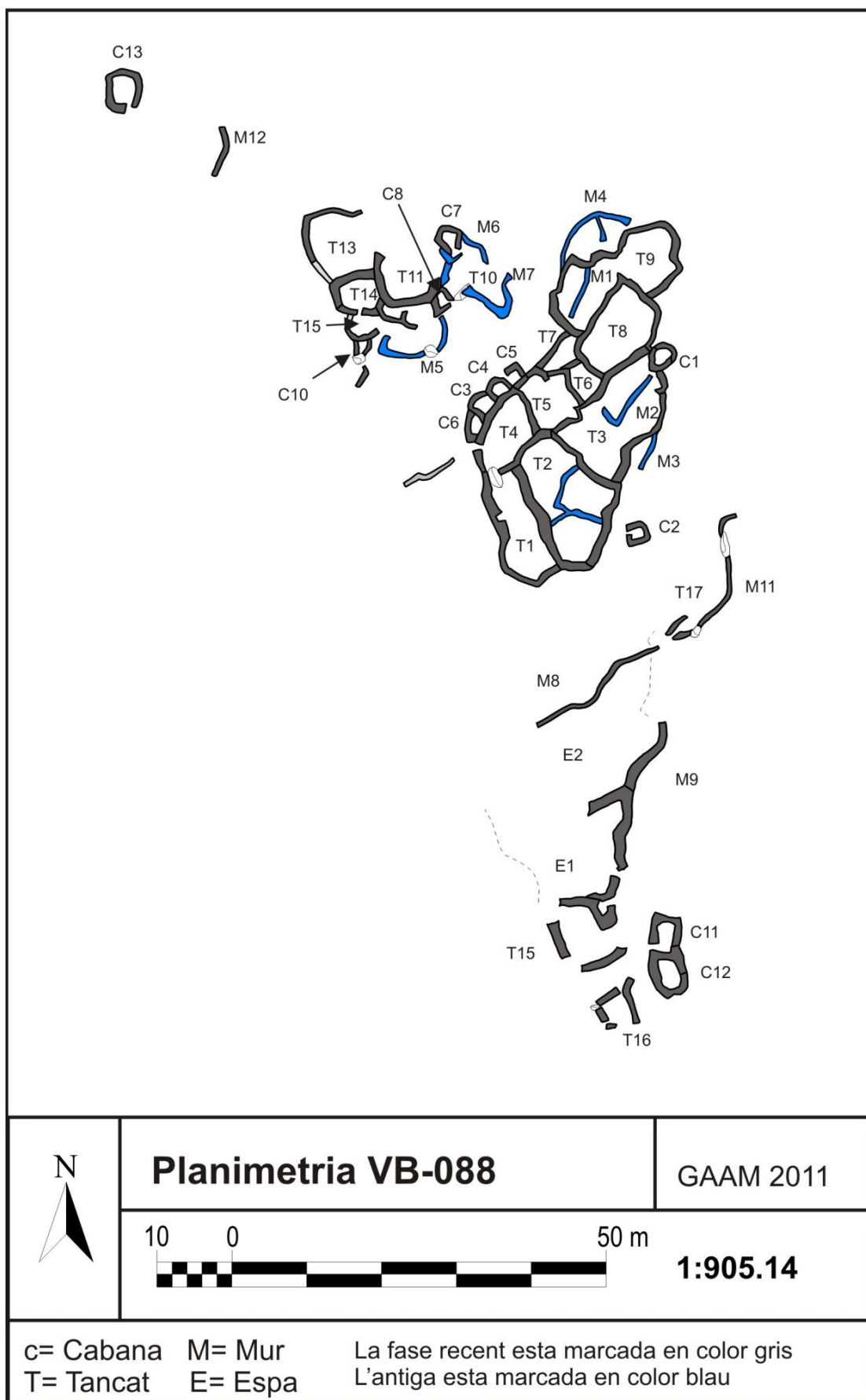
Figura 62 Aixecament topogràfic del conjunt VB-088.
