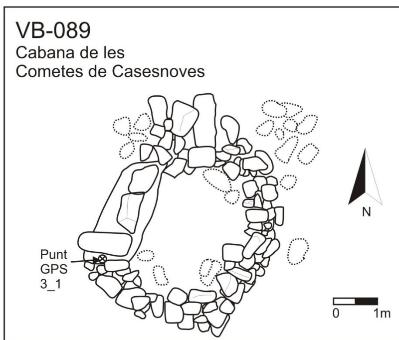
Figura 48: Croquis a escala de la cabana VB-089
