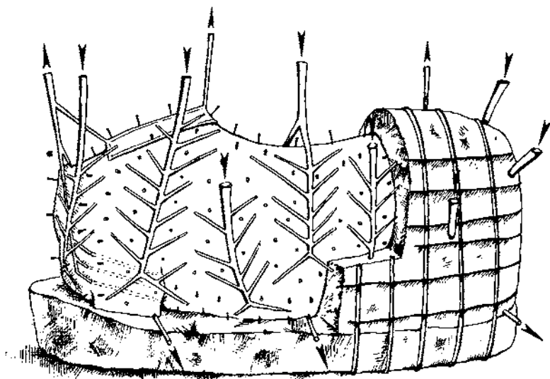
Fig. 4. Ricostruzione ipotetica dei canali di drenaggio (scolatoi, sfiatatoi e canali di getto) di un tronco di Cavallo di San Marco. In tratteggio sono gli sfiatatoi interni. Ben visibili sono pure i chiodi-distanziatori che stanno su tutto il corpo. Sopra il modello sta un mantello di materiale refrattario cerchiato in ferro.
