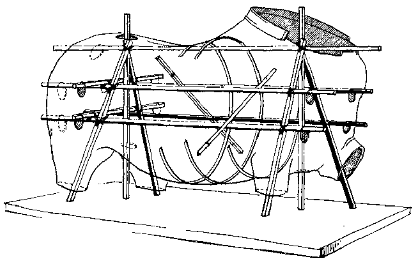
Fig. 3. L'armatura interna di un tronco di Cavallo di San Marco: sui due treppiedi di sostegno sono legati tanti lunghi perni in posizione orizzontale. Su questi stanno obliquamente numerosi distanziatori a sezione triangolare.
