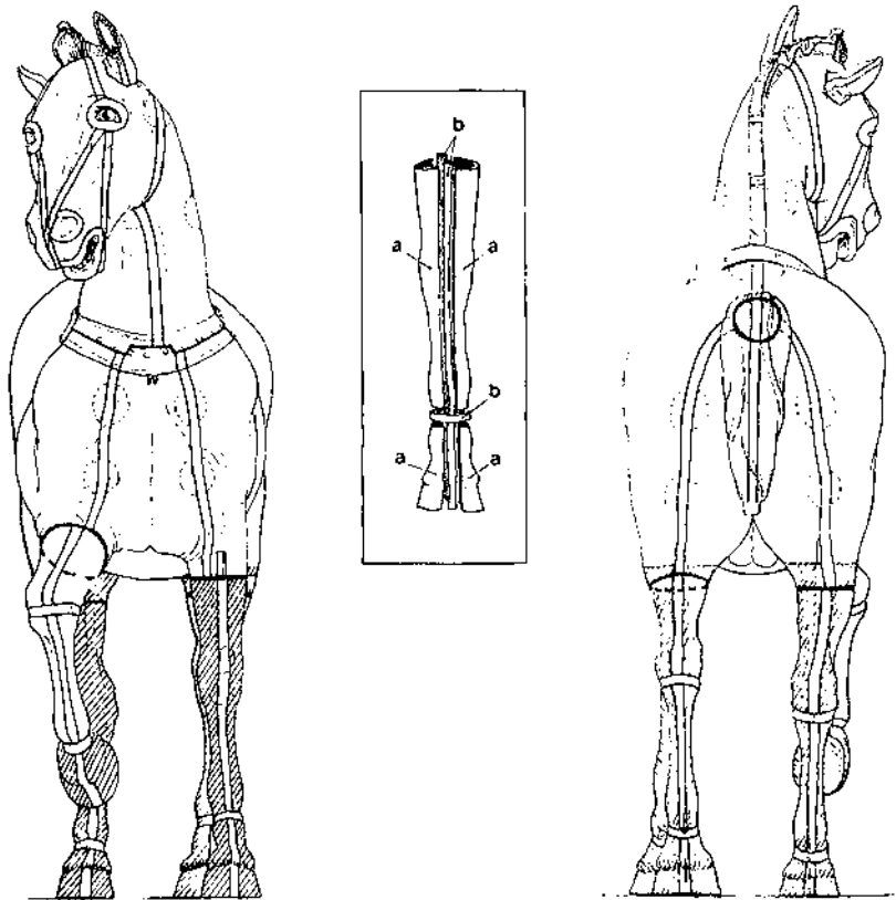
Fig. 2. I tasselli concavi o scorzoni congiunti da nastri di cera nella parte anteriore e posteriore di un Cavallo di San Marco (qui il B); le zampe, fuse a parte, sono poi state riempite di piombo per una altezza media che è stata indicata con il tratteggio. Riquadro centrale: gli scorzoni (lettere a) di una zampa prima di essere uniti e saldati con i nastri (lettere b).
