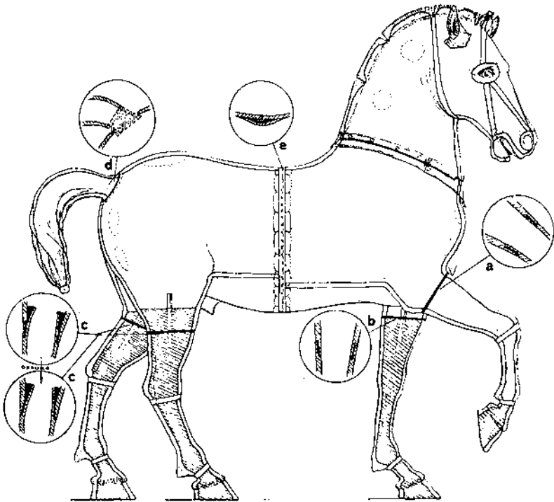
Fig. 7. I tasselli concavi o scorzoni congiunti da nastri di cera in un fianco di un Cavallo di San Marco (qui il B): attorno al tronco corre una fascia circolare data da tante «pizzette» di metallo d'apporto (rame) saldate e martellate, che venivano poste sopra il nastro di giuntura (cerchio superiore). I cerchi tratteggiati sul collo, sul petto, sulla groppa e sulle natiche indicano tante «pizze» interne di metallo poste su buchi lasciati dai perni dell'armatura. Nei cerchi fuori del corpo del Cavallo si mostrano i vari sistemi di assemblaggio delle zampe e della coda.
