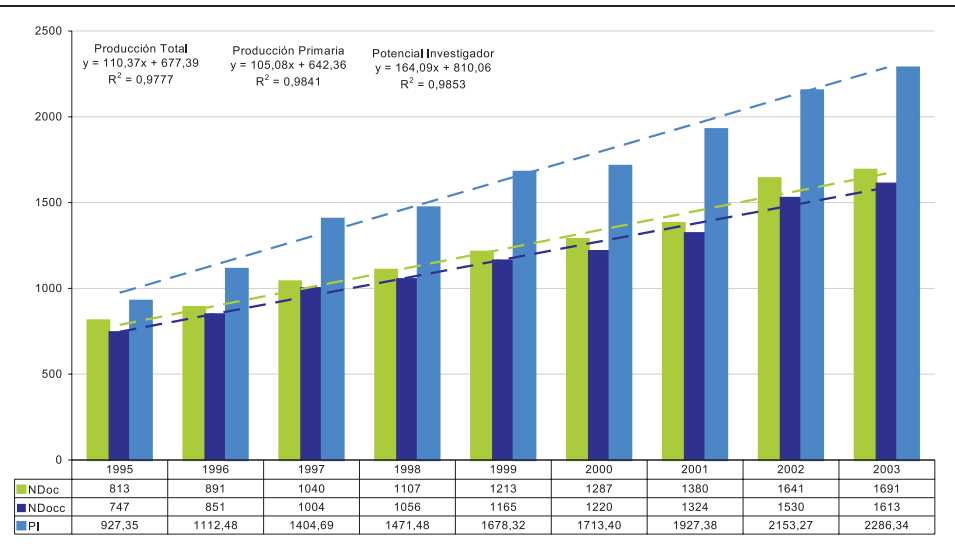
Gráfico 208. Evolución Ndoc, Ndocc y PI - Ciencias de la Tierra
