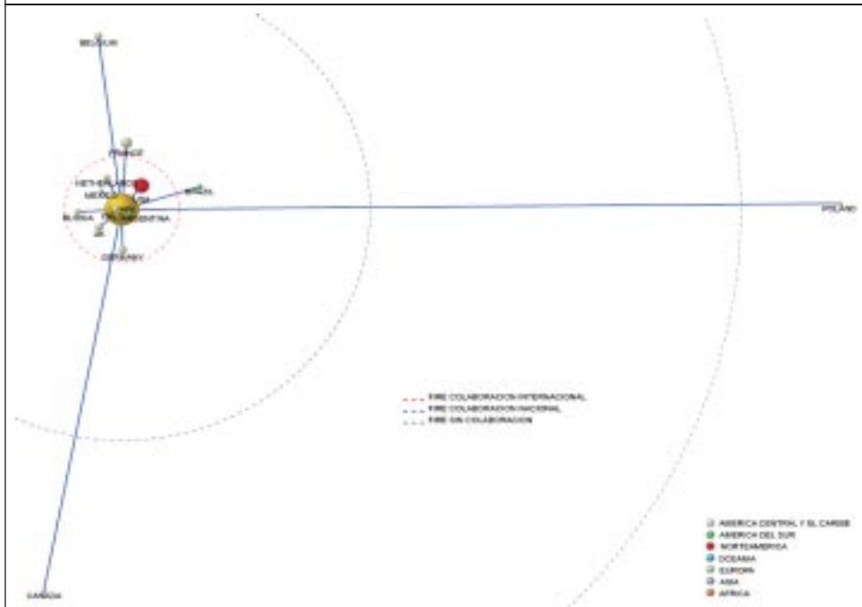
Mapa 62. Principales Países Colaboradores en Matemáticas (1995-2003)
