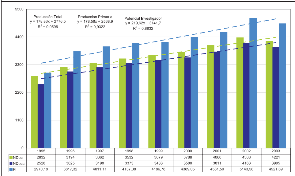
Gráfico 198. Evolución Ndoc, Ndocc y PI - Química
