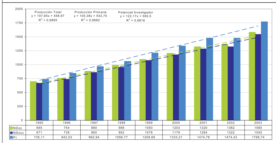
Gráfico 172. Evolución Ndoc, Ndocc y PI - Matemáticas
