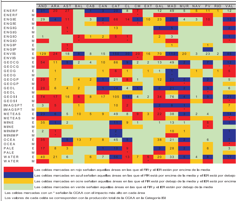
Gráfico 209. Situación de las Categorías ISI con respecto a España y al Mundo - Ciencias de la Tierra
