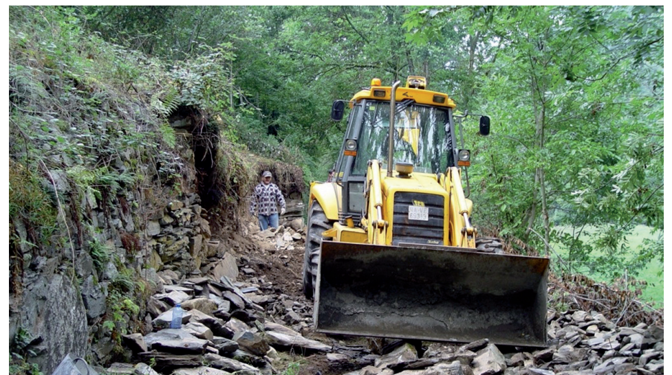
Desbrozar y rehacer las paredes, primeros pasos de la intervención en el camino.
