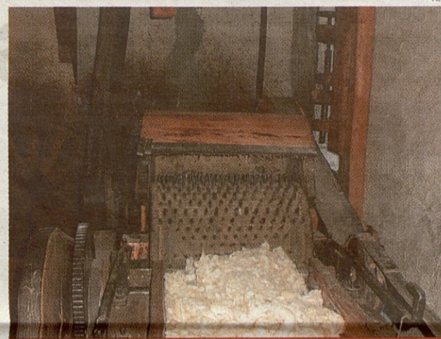
Una de las máquinas expuestas en la Fabrica dera Lan.
