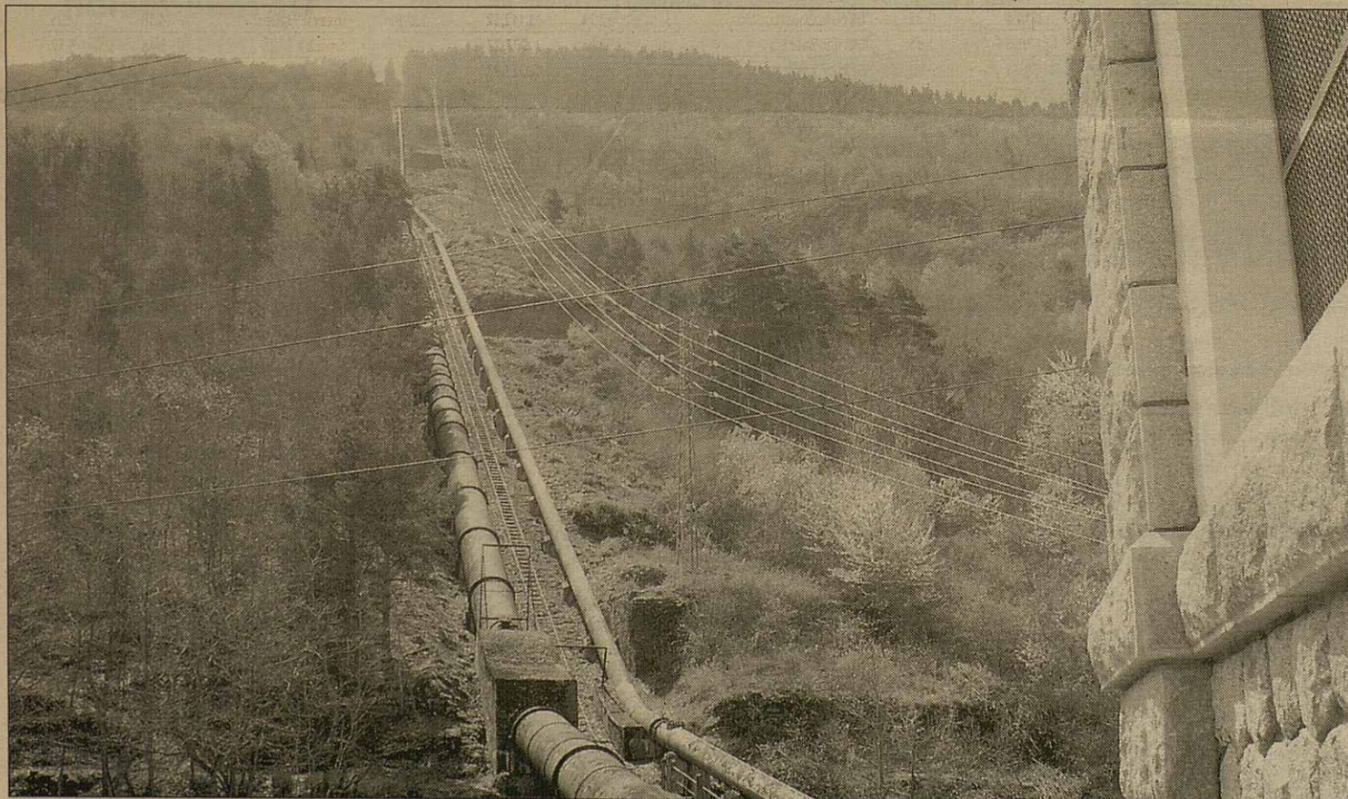
Es canalizacions d'aigua dera centrau de Benós en terçon de Lairissa
