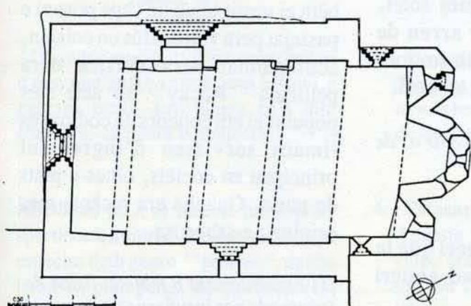
Planta glèisa St. Estèue de Betren (Catalunya Romànica).
