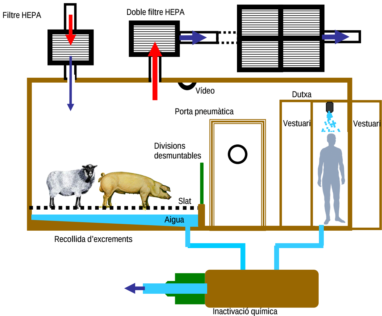
Fig.1. Disseny esquemàtic del box experimental.
