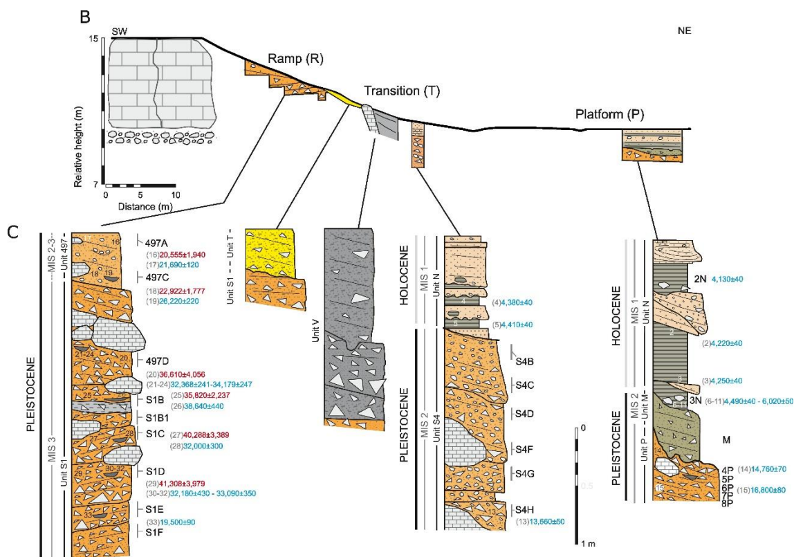
Figura 8.- Seqüència estratigràfica de la Cova Gran de Santa Linya: Crono-estratigrafia dels sectors R, T i P. Llegenda: 1) Substrat, 2) Àrees excavades, 3) Corbes de nivell (0,5 m), 4) Transsecte longitudinal NE-SW, 5) Drenatge, 6) Blocs calcaris, 7) Sorres, 8) Dipòsits d'estabulació, 9) Argiles i sorres, 10) Argiles, sorres i llims, 11) Clastes arrodonits i subarrodonits, 12) Clastes angulars i subangulars, 13) Blocs, 14) Carbonatació, 15) Estratificació, 16) Discontinuitat, 17) Fogars, 18) Datacions TL, 19) Datacions 14C AMS, 20) Unitats estratigràfiques, 21) Nivells arqueològics, 22) MIS. Modificat de Mora, et al. 2011.
