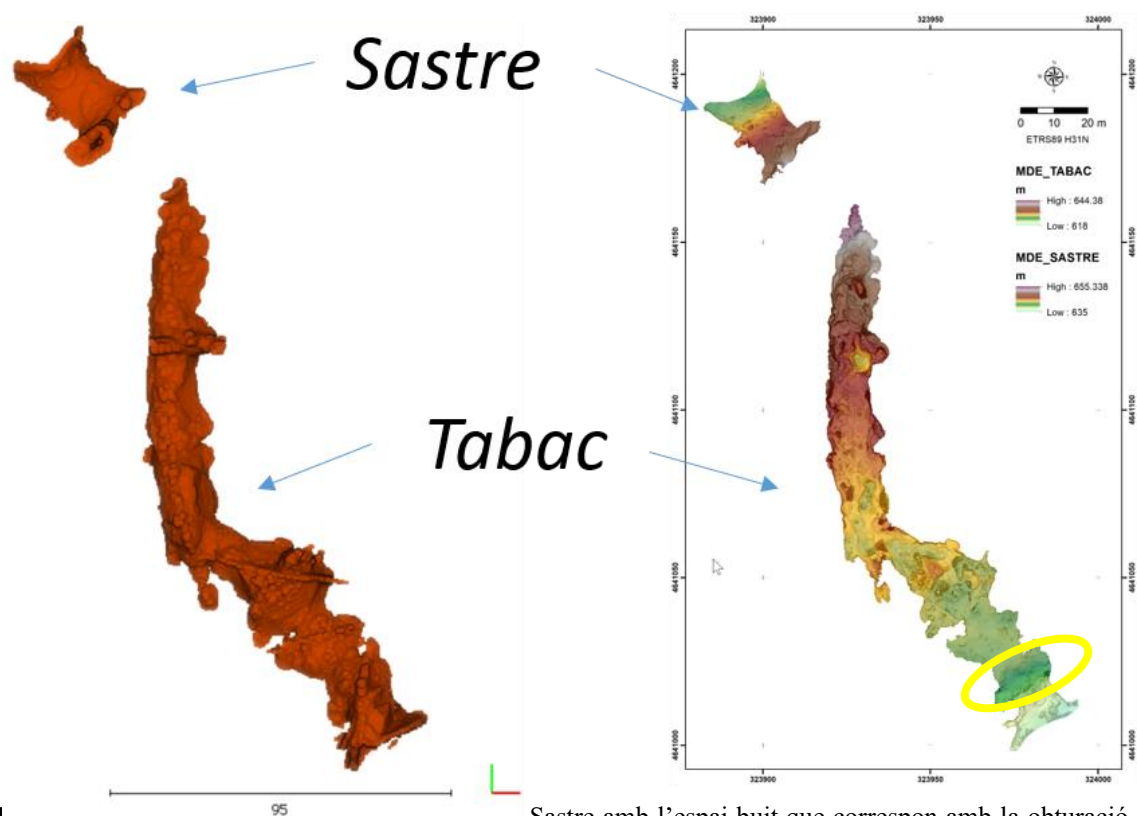
Figura 6. Model 3D dels cavitats Tabac i de Sastre amb l'espai buit que correspon amb la obturació entre ambdues cavitats. En groc correspon amb la sala el·lipsoidal on s'estan portant a terme les excavacions arqueològiques.
