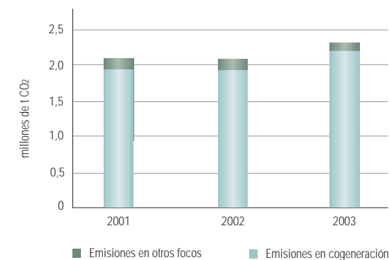
Emisiones CO 2 ENCE (según el tipo de emisión)
