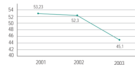
Evolución del consumo de agua en la producción de celulosa (m 3 /t celulosa)
