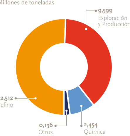
EMISIONES DE CO 2 POR ACTIVIDAD
