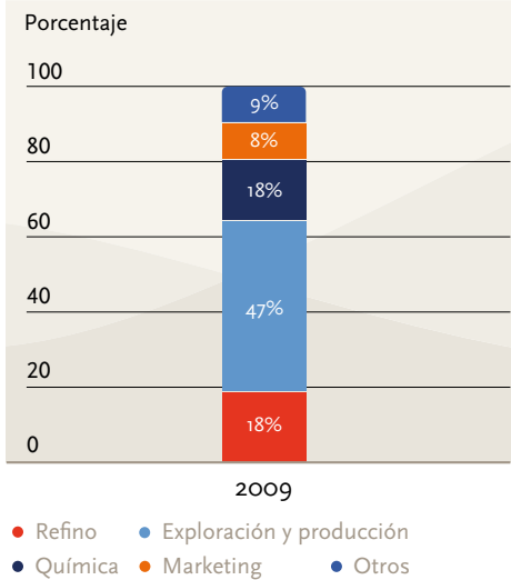
EMISIONES DE COVNM POR ACTIVIDAD
