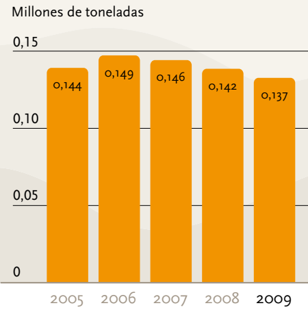
EMISIONES DIRECTAS DE CH 4 (2)
