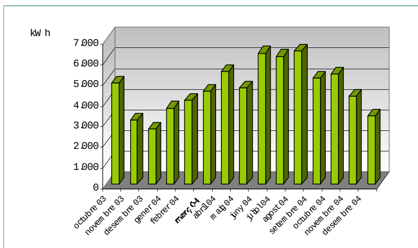
Producció elèctrica de la central fotovoltaica
