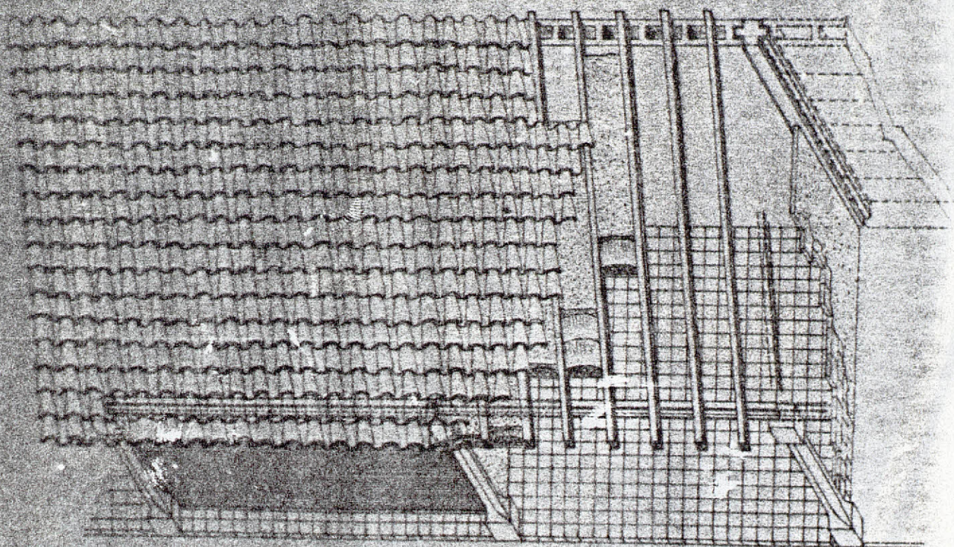
DETALL DE CONSTRUCCIÓ D'UN MÓDUL PORXAT
