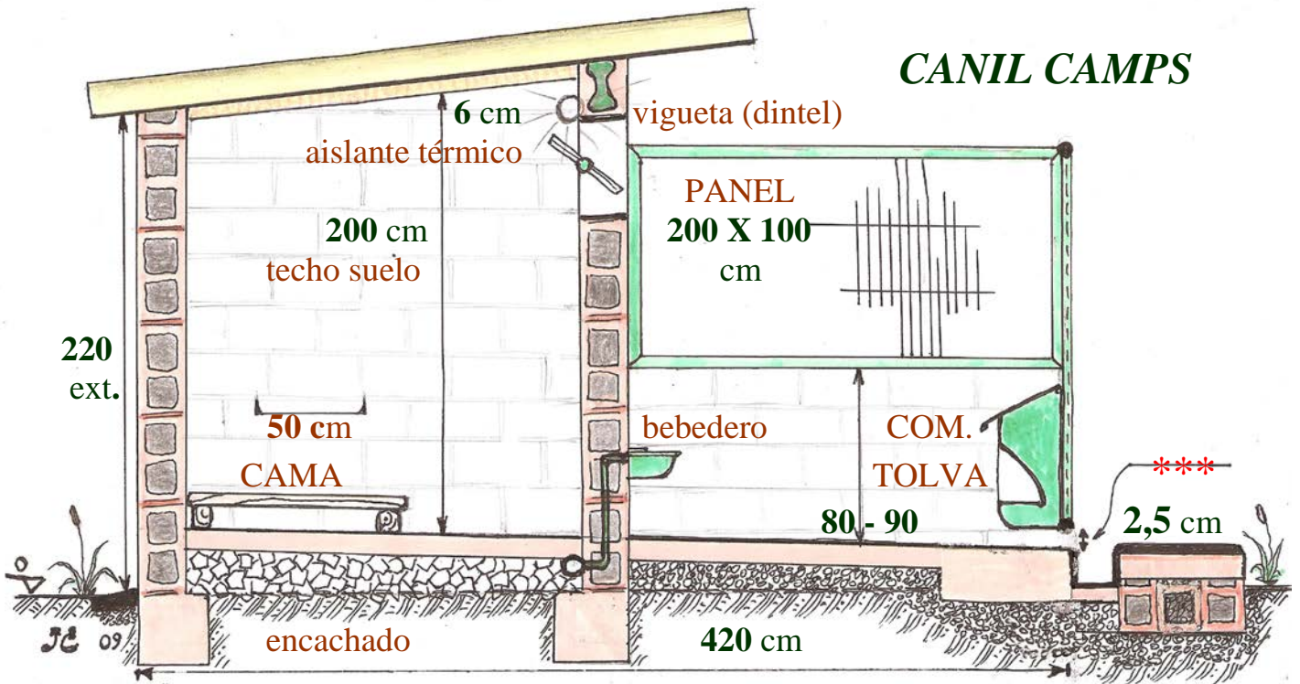
ALZADO
