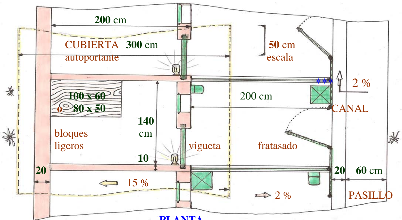
PLANTA
