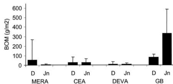
Figure 4. Benthic organic matter (BOM) for the three Atlantic streams and for the Mediterranean stream (GB). The graph shows mean values ( \pm 1 SE). D = December samples; Jn= June samples. Materia orgánica bentónica (MOB) para los 3 ríos atlánticos y el río mediterráneo (GB). Los gráficos muestran los valores medios ( \pm 1EE). D = muestras de diciembre; Jn= muestras de junio.
