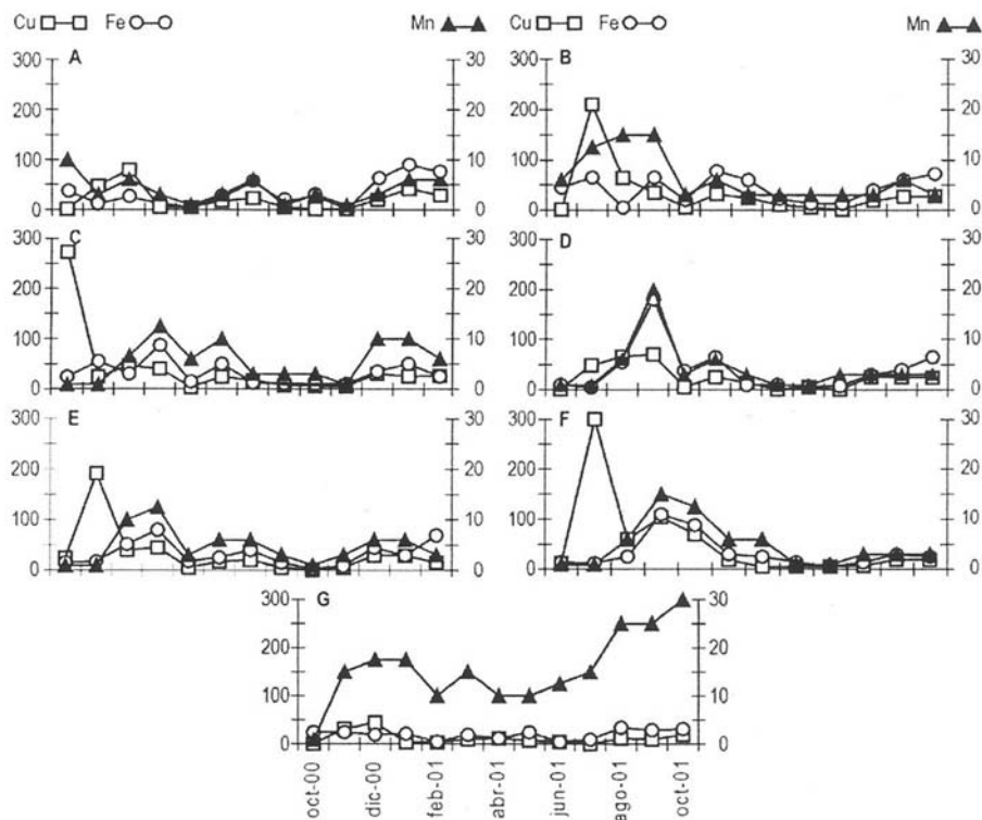
Figura 4. Variación anual de las concentraciones de cobre, hierro y manganeso ( \text{mg/l} \cdot 10^2 ): A-R. Blanquito; B-R. Churqui; C-R. de Las Carreras; D-R. de La Ovejera; E-R. Tafi; F-R. El Mollar y G-R. Los Sosa. Annual variation of copper, iron, and manganese concentrations ( \text{mg/l} \cdot 10^2 ): A-R. Blanquito; B-R. Churqui; C-R. de Las Carreras; D-R. de La Ovejera; E-R. Tafi; F-R. El Mollar and G-R. Los Sosa.
