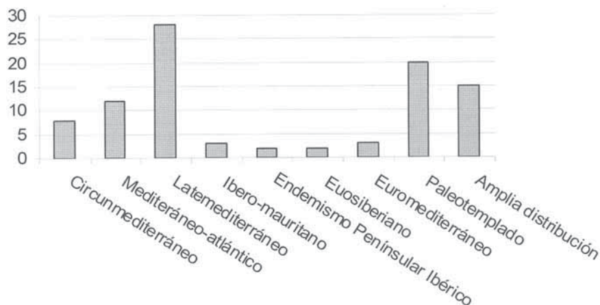
Figura 3. Elementos fitogeográficos en el área de estudio. Phytogeographical elements in the study area.
