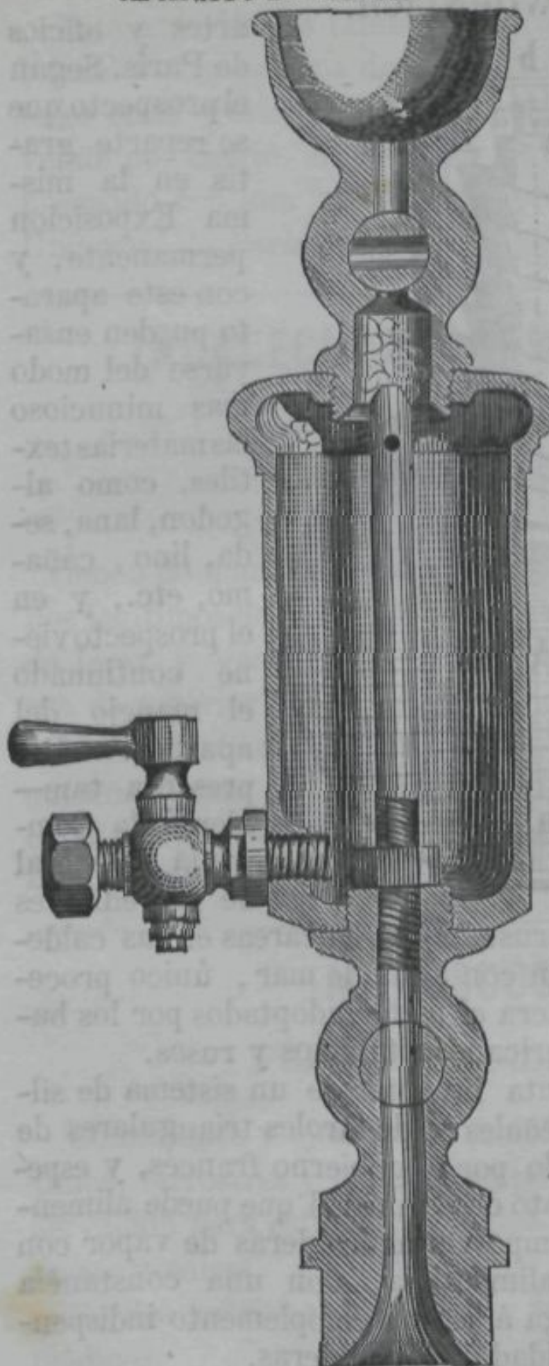
Corte.
