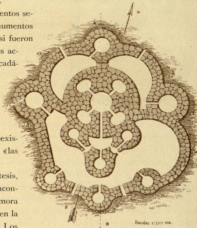
Fig. 121. - NURAGHE DE ORTU. - PLANTA, SEGÚN LA MÁRMORA
