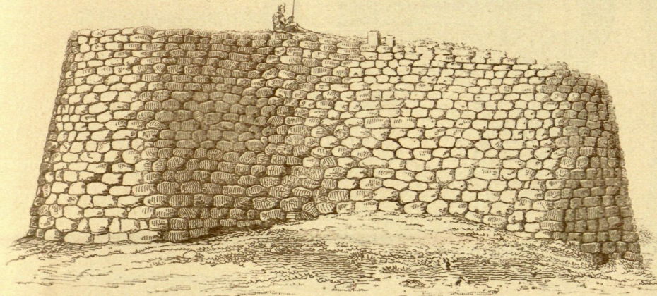
Fig. 117. - NURACHE DE LOSA. - ALZADO, SEGÚN LA MÁRMORA
