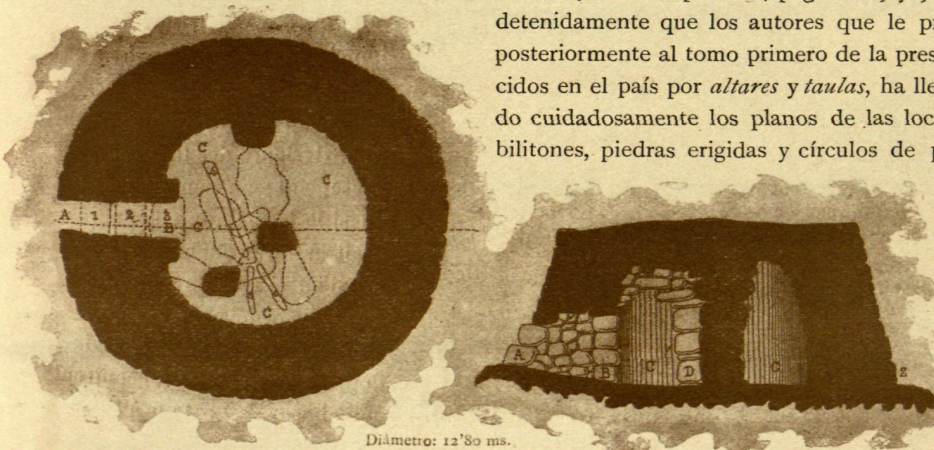
Fig. 130. - TALAYOT DE S' AGUSTÍ, CERCA DE ALAYOR (MENORCA), SEGÚN CARTAILHAC
