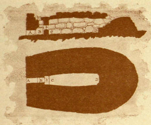
Fig. 137. - NAVETA DE RAFAL RUBÍ, SEGÚN CARTAILHAC
