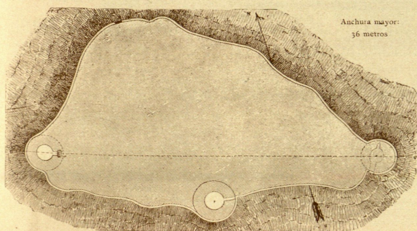
Fig. 122. - NURAGHE DE SARECCI. - PLANTA, SEGÚN LA MÁRMORA ARQUITECTURA
