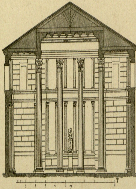
7 Basílica de Pompeya
