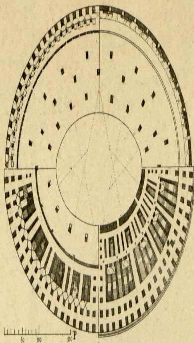
1 Planta del Colosseo
