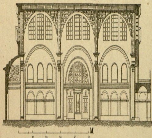
8 Basílica de Constantino (sección)
