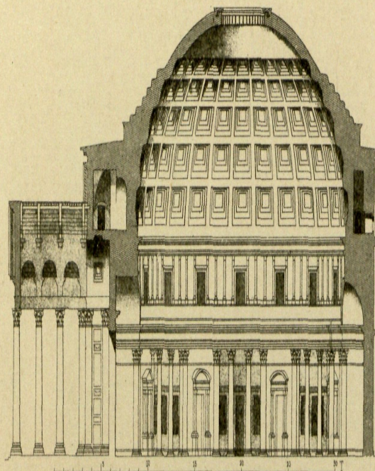
4 Panteón (sección)
