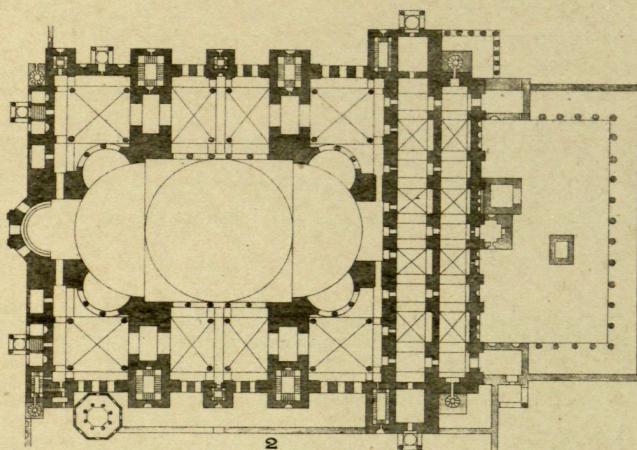
2 Planta de la fig. 1
