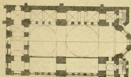
6 Planta de la fig. 4.
