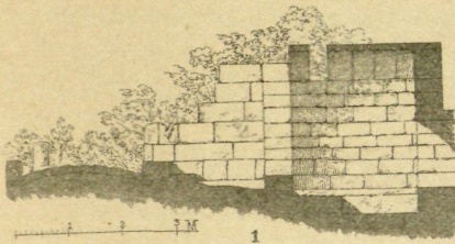
1 Casa del manantial en Tusculum
