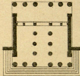
Planta de la fig. 14
