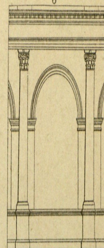
5 Arcadas del Colosseo
