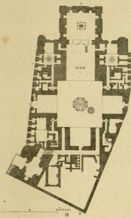
Planta de la fig. 2
