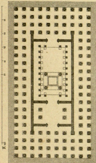
2 Planta de la fig. 1
