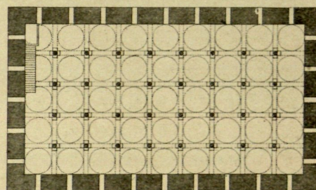
5 Cisterna en Constantinopla (Planta)
