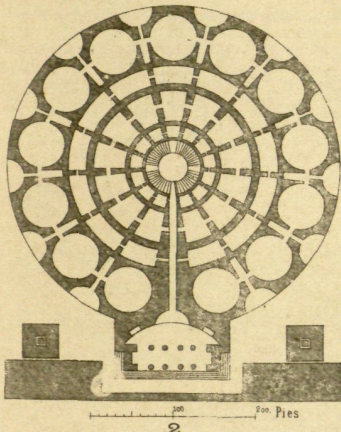
2 Mausoleo de Augusto (planta)
