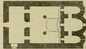
4 Planta de la fig. 3
