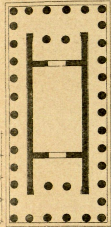
Planta de la fig. 1
