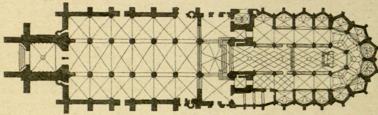
3 Cat. de Friburgo planta
