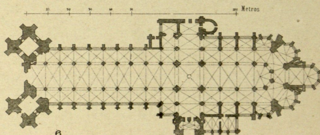
6 St. Ouen de Ruan.—Planta
