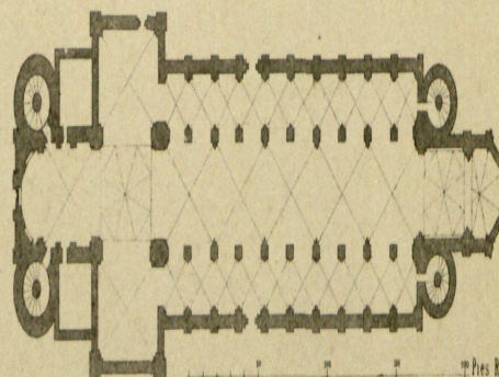
Planta de la catedral de Worms
