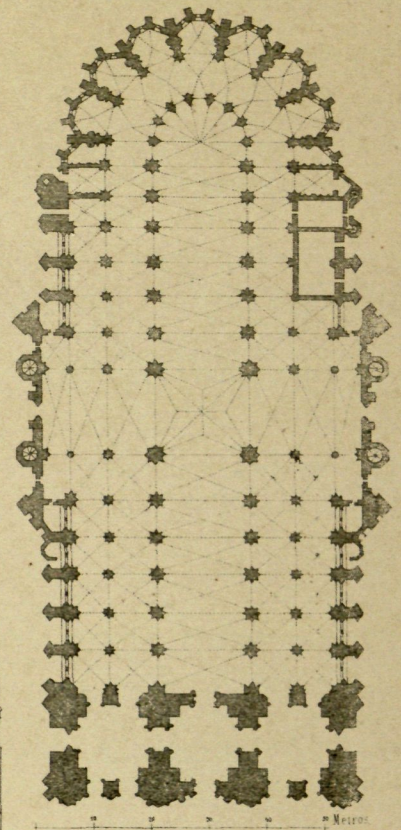
3 Catedral de Orleans Planta
