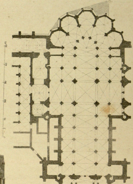
6 Catedral de León
