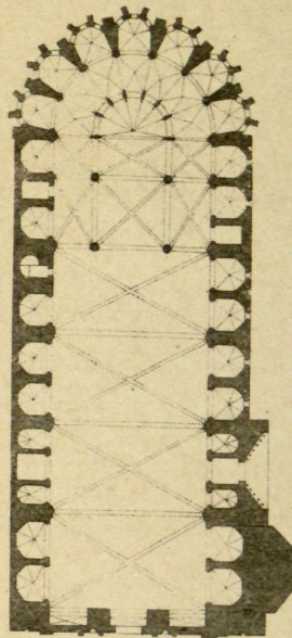
8 Catedral de Gerona
