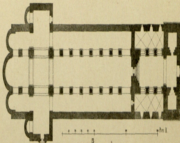
Planta de la fig. 4
