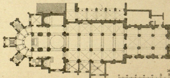
6 San Filiberto Tournus
