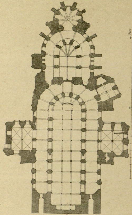
2 Catedral de Cantorbery (planta de la cripta)
