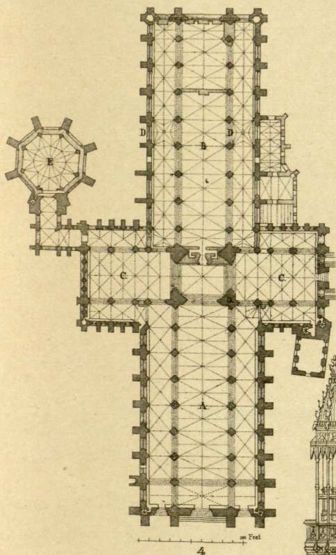
4 Planta de la Catedral de York
