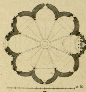
San Miguel d'Entraigues
