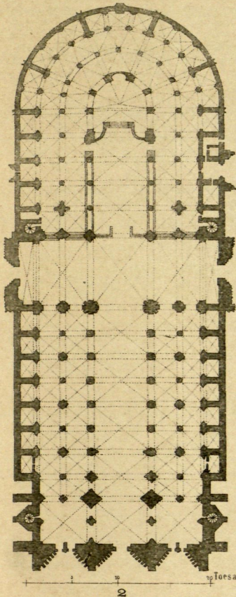
2 Planta de Nuestra Señora de París
