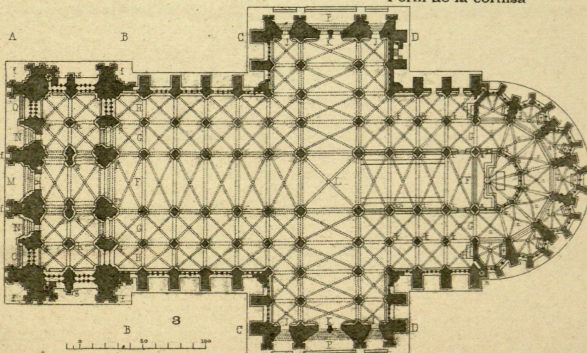
3 Cat. de Colonia. Planta
