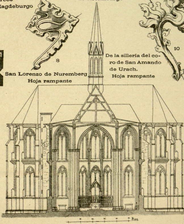
2 Sección de la iglesia de Santa Isabel en Marburgo
