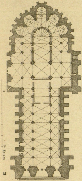
Catedral de Reims.—Planta
