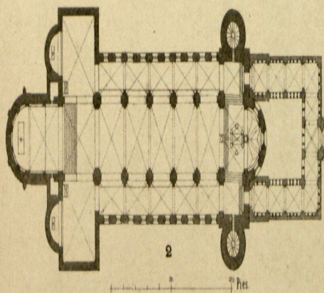
Planta de la fig. 1
