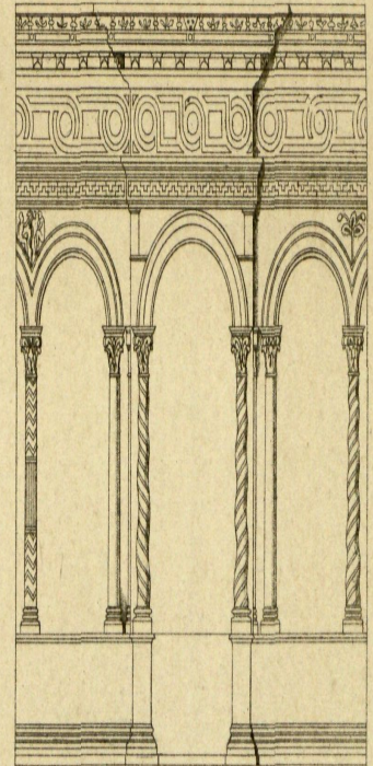
5 Arcos del claustro de San Pablo de Roma
