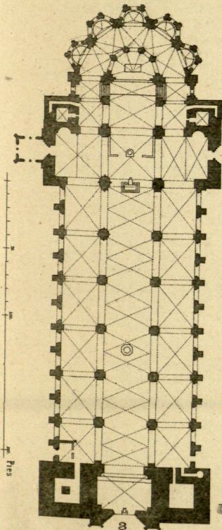
3 Cat. de Magdeburgo. Planta
