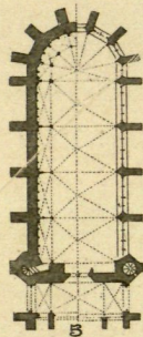
3 M. Planta de Nuestra Señora de París
