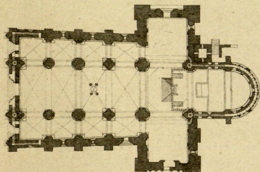
8 Planta de la fig. 2
