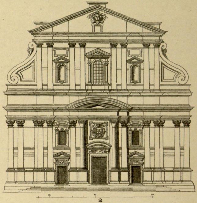
Fachada de la iglesia del Gesù en Roma (G. della Porta)
