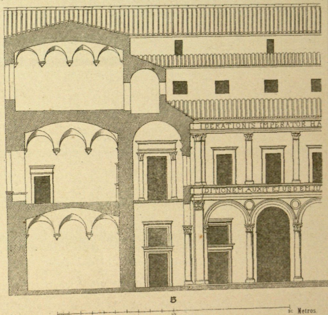
Palacio de Urbino
