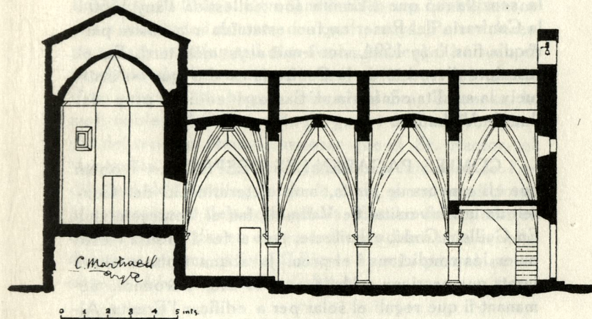
Secció longitudinal de l'Ermite del Roser, de Vallmoll
