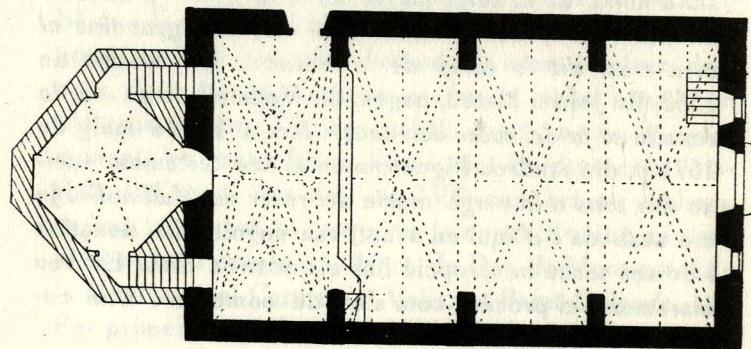
Planta de l'Ermita del Roser de Vallmoll. La part ratllada indica l'obra moderna del Cambril, del segle passat.
