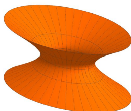
Hiperboloïde d'un full \left(\frac{x}{a}\right)^2 + \left(\frac{y}{b}\right)^2 - \left(\frac{z}{c}\right)^2 = 1
