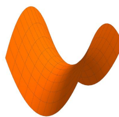
Paraboloïde hiperbòlic \left(\frac{x}{a}\right)^2 - \left(\frac{y}{b}\right)^2 = cz
