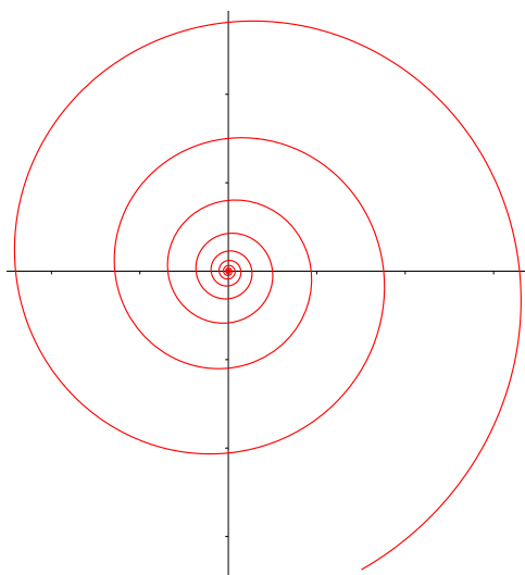
Espirale logarítmica amb a = 1 , b = -0.1 i t \in [-20, 100] .
