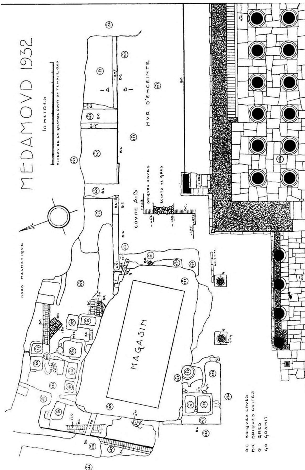
PLANO 22: Plano de la excavación alrededor del almacén sur al Noroeste del templo en 1932 (BISSEON DE LA ROQUE 1933: pl. VI).
