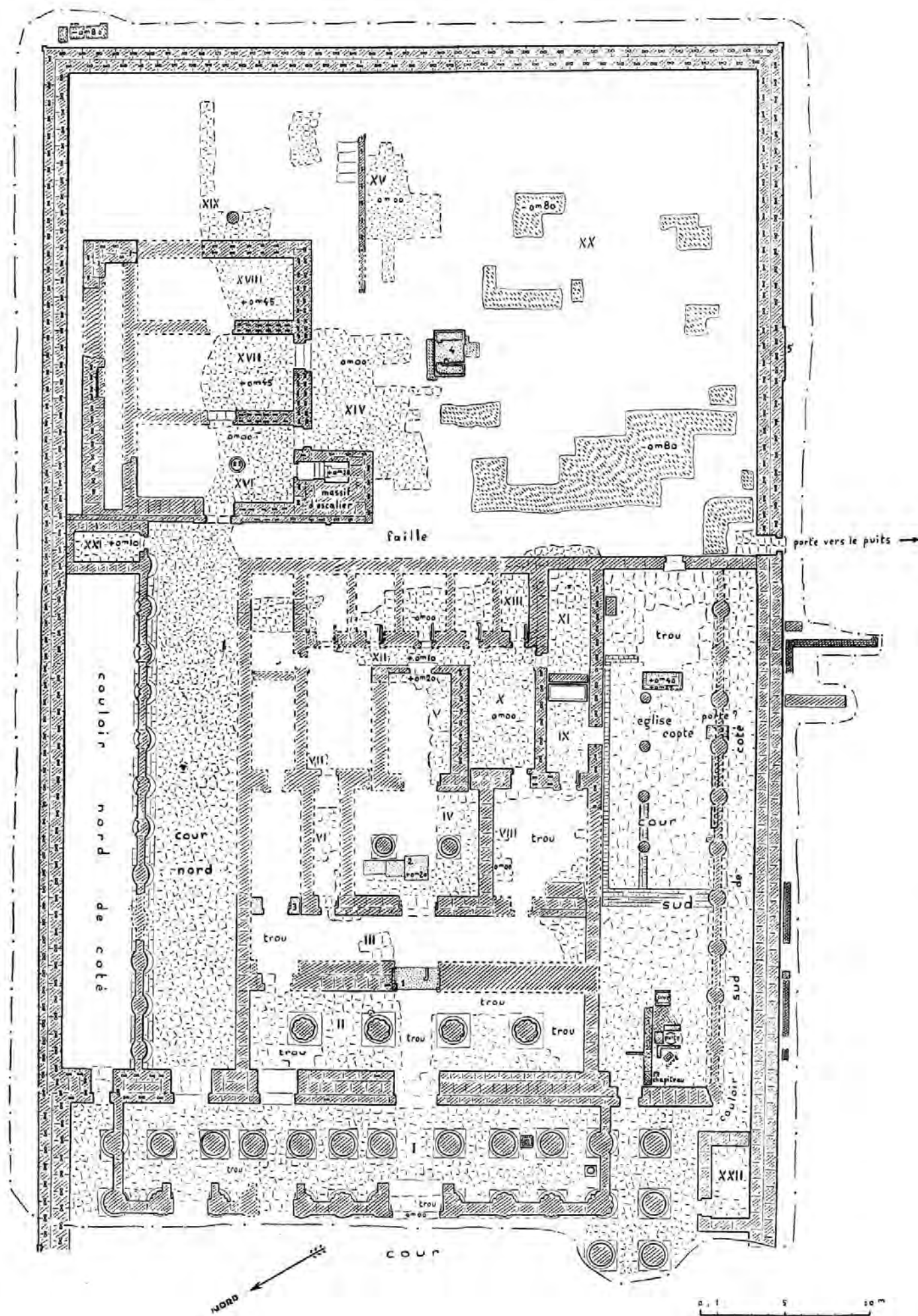
PLANO 3: Plano del templo en 1925, con las estructuras conservadas y restituídas (BISSEON DE LA ROQUE 1926: pl. III).
