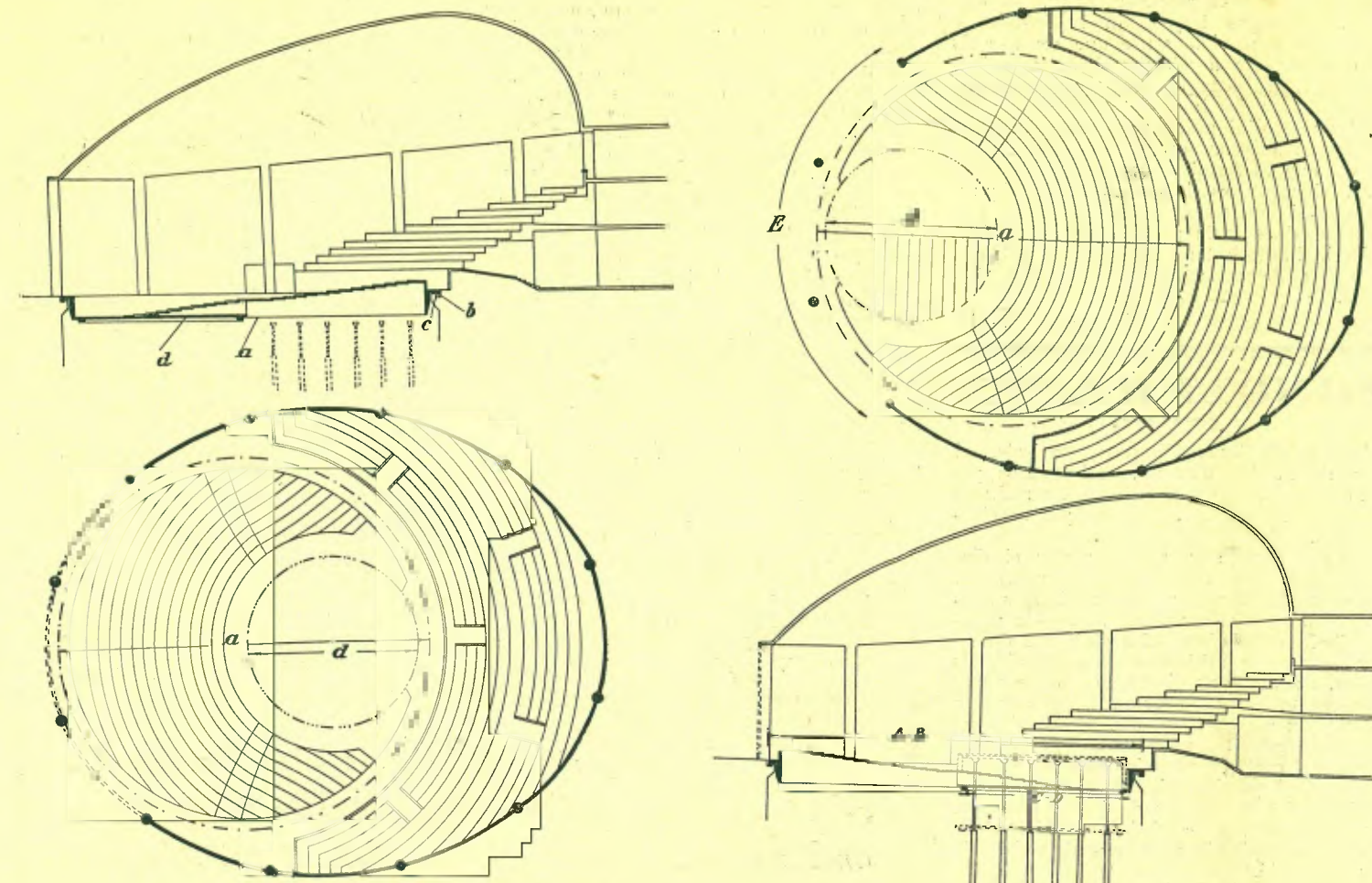
Els gràfics primer i quart mostren seccions longitudinals del teatre; els segon i tercer, el pla del teatre en dues posicions diferents de l'escenari giratori. a, disc giratori, en part ocupat per seients, sobre el qual el disc d, que es pot alçar i abaixar en sentit perpendicular, pot servir també de prosceï o, posant-hi seients, complementa el pati en les representacions amb l'escenari corrent
