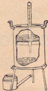
BAÑO-MARÍA para 12 ensayos
