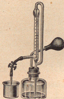
ACEDIMETRO «DORNIC»
