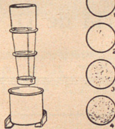
FILTRO RECORD para determinar el grado de impureza de la leche
