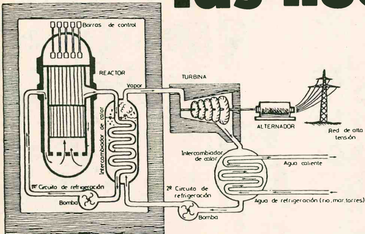
Esquema de una central nuclear
