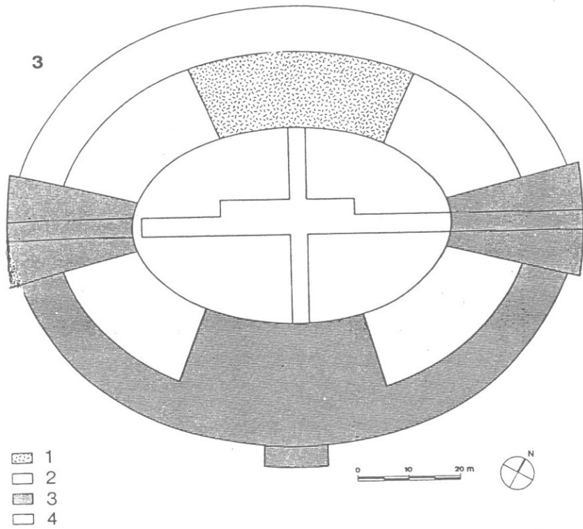
Fig. 163 - Planta esquemàtica de les tècniques constructives utilitzades en l'Amfiteatre. 1: Estructures tallades a la roca, 2: Estructures massisses, 3: Estructures construïdes, 4: Estructures massisses o construïdes.
