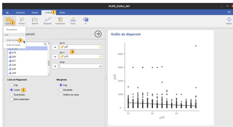
Imatge 134. Diagrama de dispersió o XY amb jamovi.
