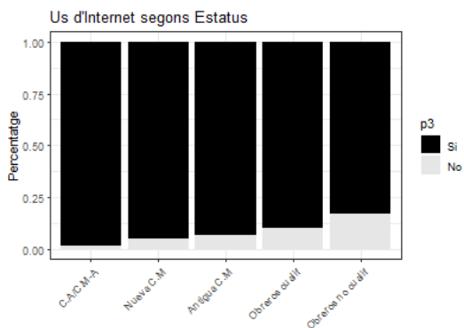
Imatge 106. Representació gràfica de taula de contingència (MILLORADA)
