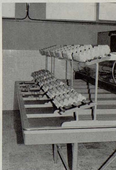
Detalle de la mesa de recogida, con repisas para colocación de bandejas vacías y llenas
