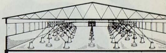
Detalle de una instalación de comedero automático PUIG COLGANTE y BEBEDEROS DRINKEVE. Se pueden instalar 1, 2 y 3 filas de tolvitas PLASTIC PUIG o PUIG-MATIC, filas se doblan con las ventajas de la distribución de pienso y retorno.
