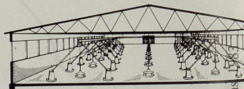
Detalle de una instalación de comedero automático PUIG COLGANTE y BEBEDEROS DRINKER Se pueden instalar 1, 2 y 3 filas de tolvas PLASTIC PUIG o PUIG-MATIC , se doblan con las ventosas distribución de pienso retorno.
