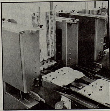
5. Nuevo sistema de desapilado con control electrónico de estuches y cartones que permite una máxima perfección en la operación.
