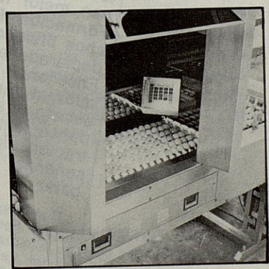
3. Control electrónico del miraje con visor digital que permite separar automáticamente los huevos defectuosos a la empacadora programada.
