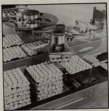
2. Nuevo sistema de succión y transferencia: mejor tratamiento de huevos con menos velocidad de movimiento.
