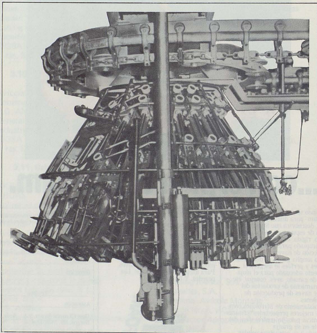
EVISCERADORA AUTOMATICA DE AVES DE ALTA PRODUCCION
