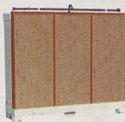
Cabina de extracción e inyección a baja velocidad con panel de celulosa. Pollos, ponedoras, reproductoras, incubadoras, etc.
