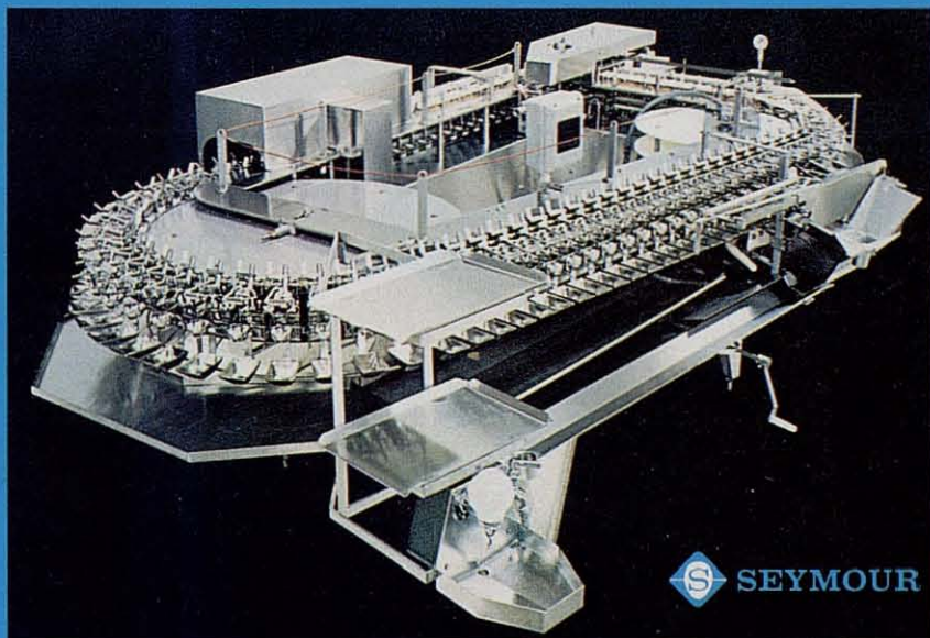
Lavadora-rompedora-separadora de huevos SEYMOUR Mod. 104 C. 36.000 huevos/h
