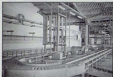
Desapilador automático
