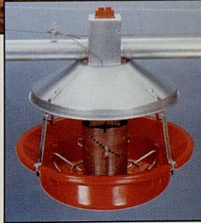
Comedero Modelo ATF™ para Pavos
