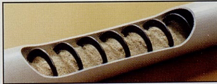
Sistema de Transporte de Alimento FLEX-AUGER®
