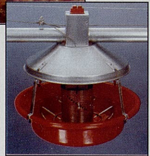
Comedero Modelo ATF™ para Pavos
