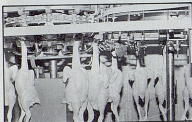
Transferencia automática
