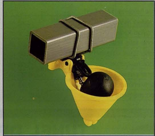
Bebederer Cazoleta M-73-92 Mixto Todas las edades
