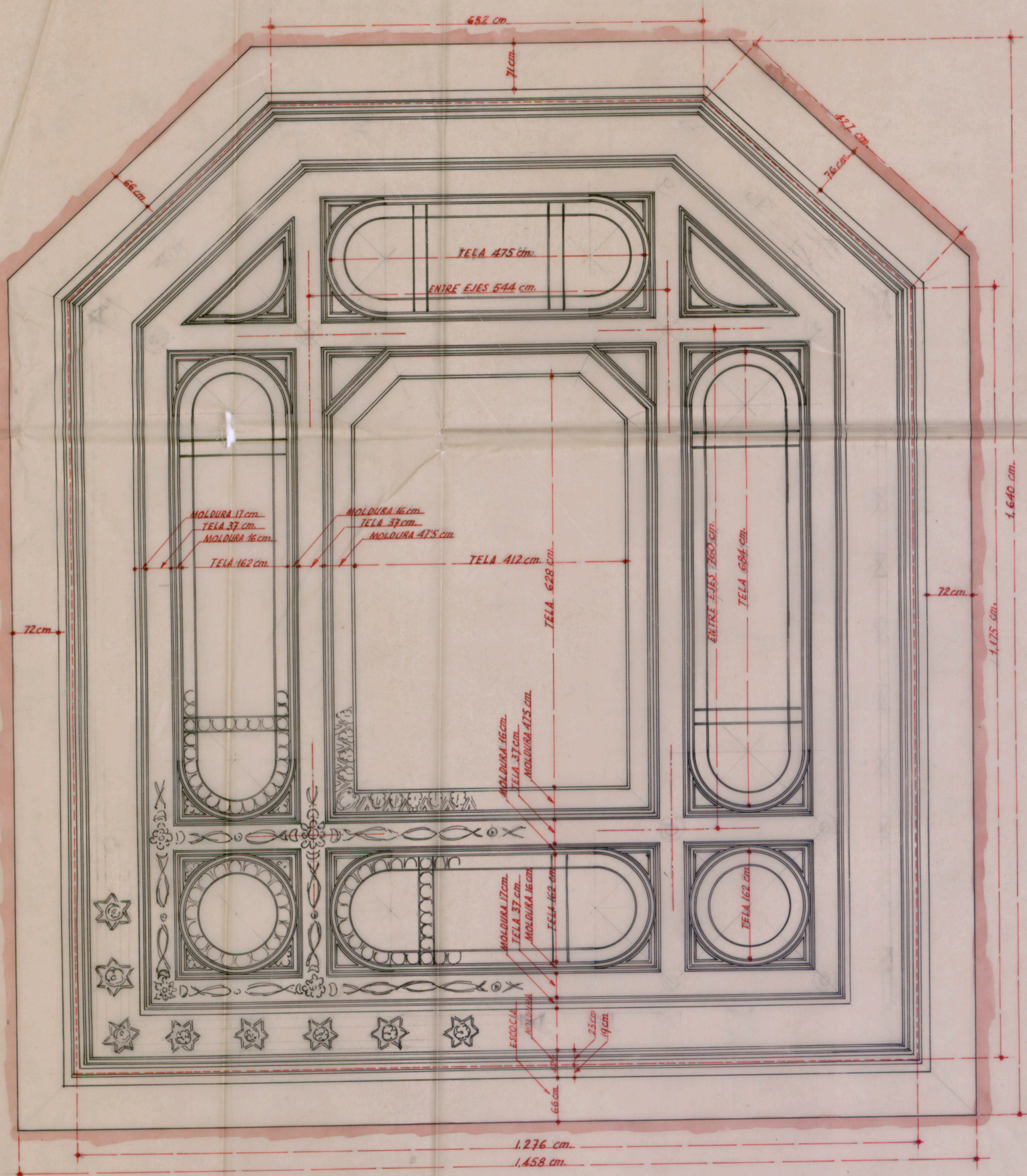
TEATRO DEL LICEO RECONSTRUCCION DEL CIELO - RASO - DEL SALON DE DESCANSO ESCALA 1:50
