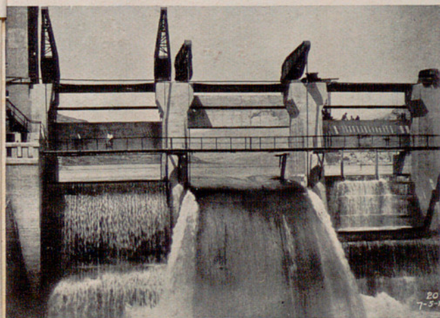
Comportes automàtiques de la Presa de Talarn (Salt de Trep, 42 500 C. V.), un dels més importants de la nostra economia hidroelèctrica
