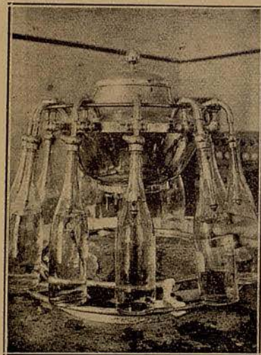
Detalle del aparato de llenar botellas
