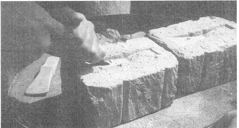
Fig. 12: Fabrication d'un moule bivalve pour haches en bronze per M. Vallesi (Italie). Journées d'Archéologie expérimentale, 1996. Cliché Ch. Chevillot.
