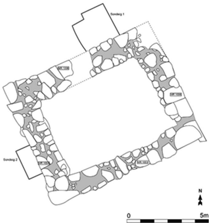
Figura 3. Plànol de les estructures de la torre de Puig d'Àlia (plànol: Carles Padrós).
