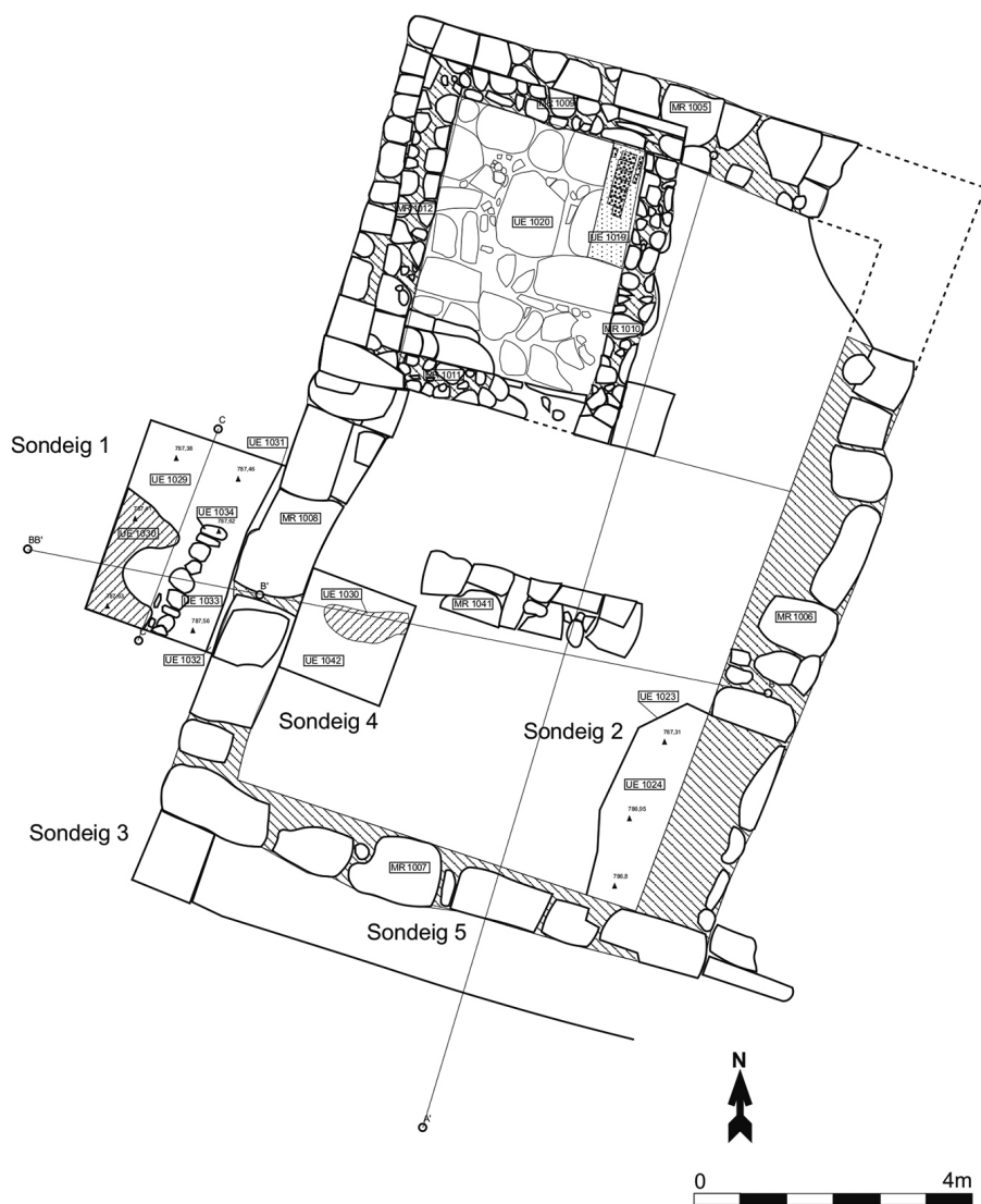
Figura 5. Tentellatge 1. Plànol final de la intervenció de l'any 2015.
